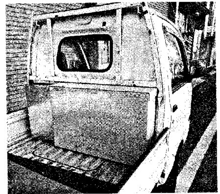
改造された軽トラの荷台に取り付けられたバッテリー
