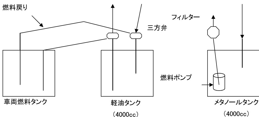
図1 燃料系統
